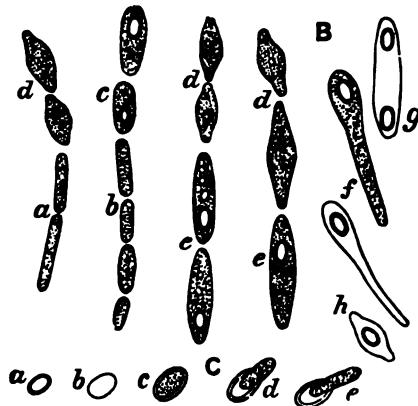
FIG. 54.— CLOSTRIDIUM BUTYRICUM , \times 1020 .
